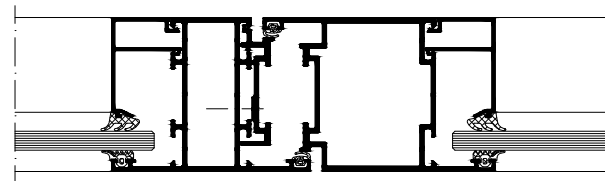
Anschlagprofil Rebate profile
