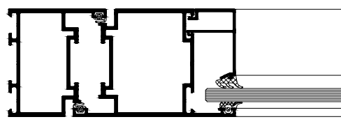
Flügelprofil Leaf profile
