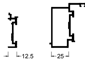
Anschlagprofil 25 Rebate profile 25
