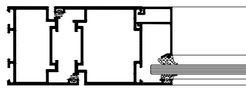
Blendrahmenprofil Outer frame profile
